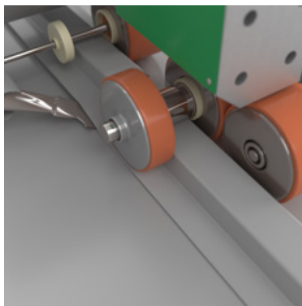
Appareil automatique de soudure à air chaud adapté grâce au kit RENOLIT ALKORSOLAR
