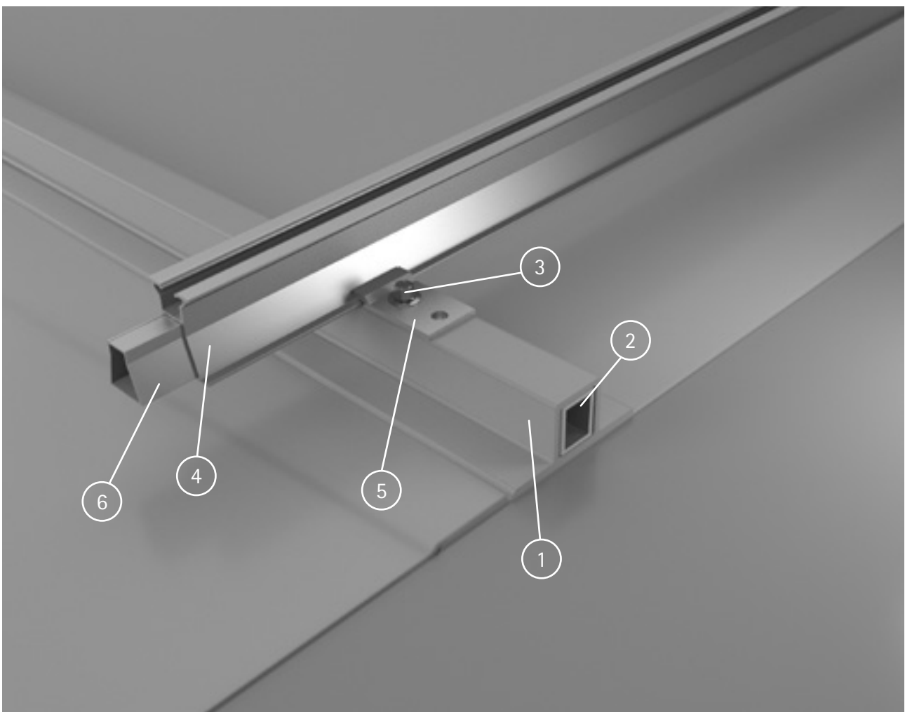
Composants du système RENOLIT ALKORSOLAR
