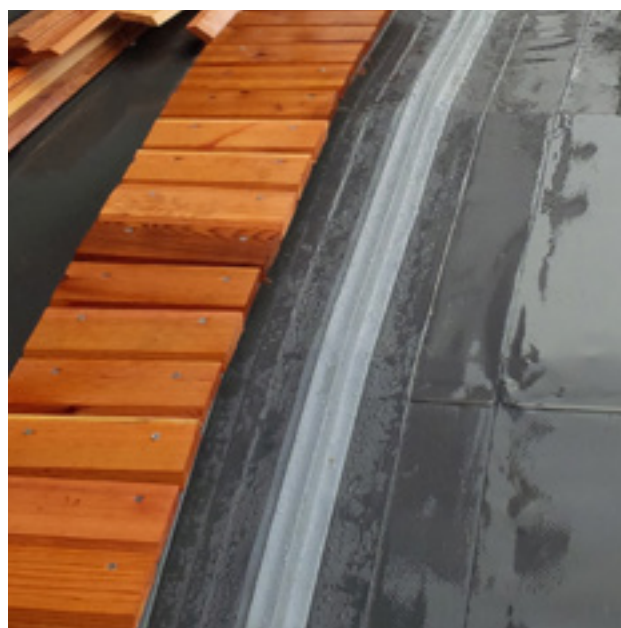
Les pièces d'habillage en bois sont fixées sur des profilés RENOLIT ALKORSOLAR
